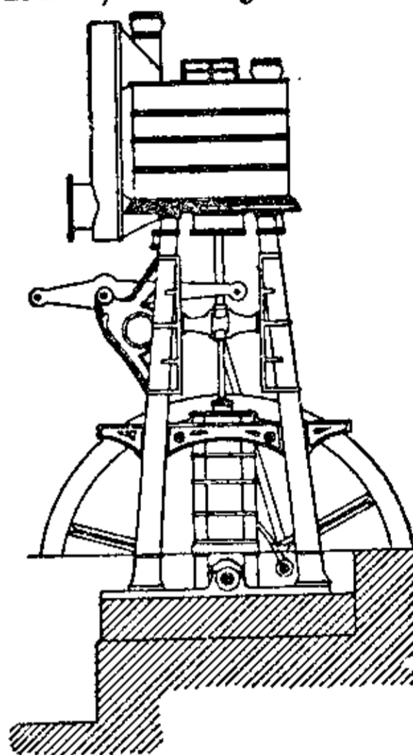
Вальцеве дувало.
