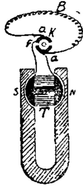
Електр. машина Сіменса з Т-якорем. Т — залізний якор, к — коммутатор, а — щітки, В — зовнішній провідник, S, N — бігуни.
