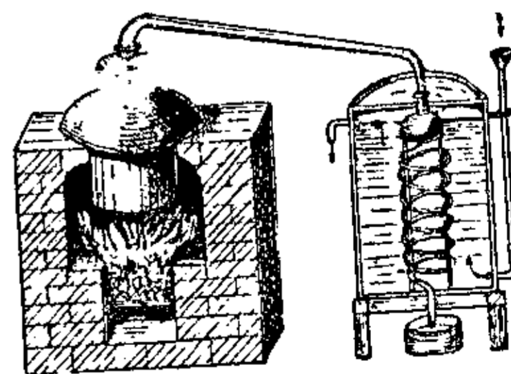
Алембик.
