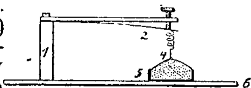
Кристалний детектор: 1. підпора, 2. пружина, 3. гвинт до наставлювання, 4. вістря, 5. кристал, 6. підпора.
