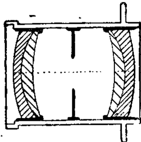
Апланат (проріз).
