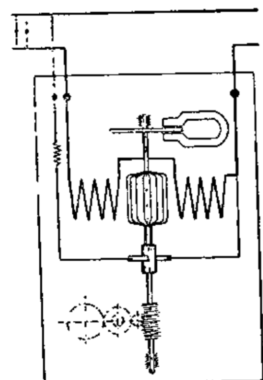
Схема двигунового електроміра.
