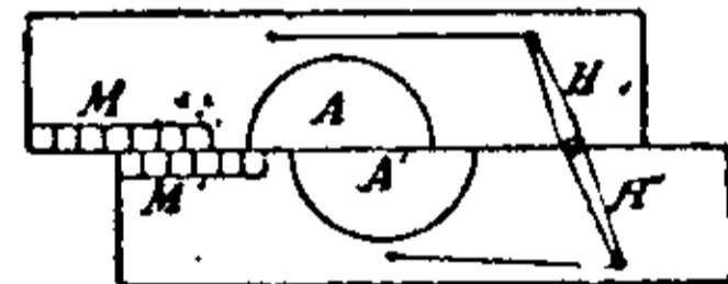
Геліометр, AA' — половина об'єктиву, NN' — підойми, MM' — мірило.
