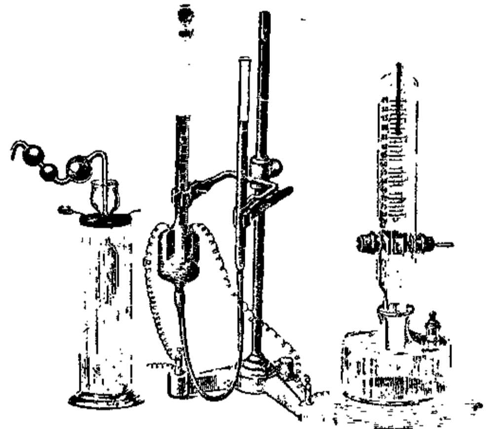
Вольтаметри з гремучим газом.
