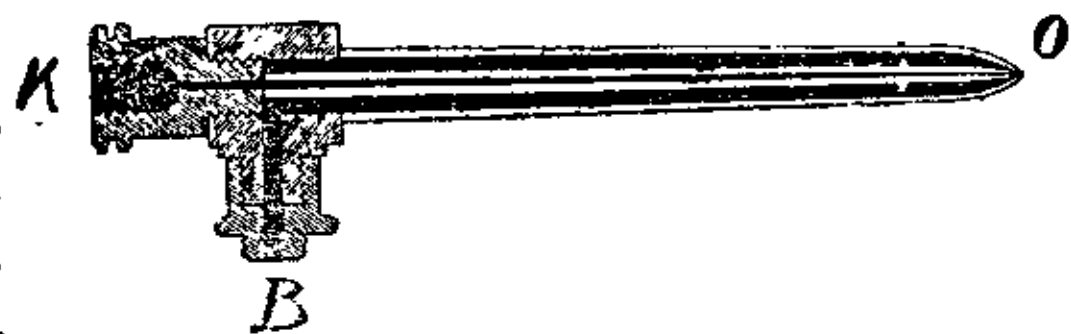
Прилад до витворення гремучого газу. К — отвір, куди йде кисень, В — отвір, куди йде водень, О — пальник.
