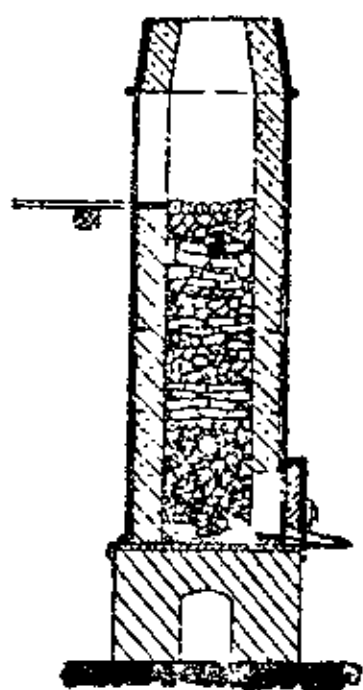
Вагранка.
