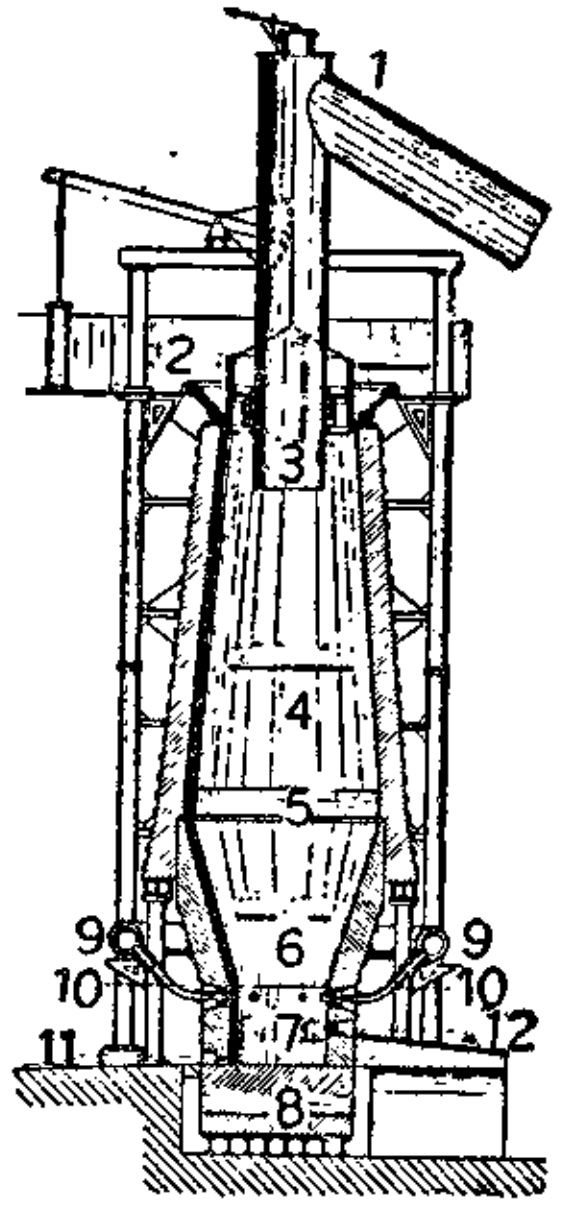
Доменна піч. 1. 3. рури, якими відводять газу, 2. поміст, на якому довозять вугілля, 3. отвір, яким насипається руда і кокс, 4. 5. 6. піч, в якій витоплюється залізо, 7. збірник розтопленого заліза, 8. спід печі. 9. 10. рури, якими вдувається гаряче повітря, 11. отвір, яким витікає розтоплене залізо, 12. отвір, яким виходить жужіль.
