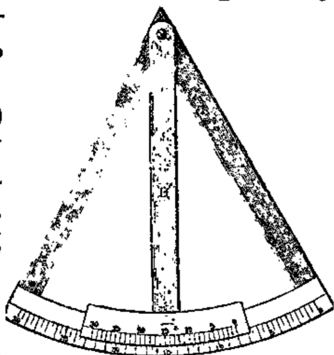
Верньєр коловий.
