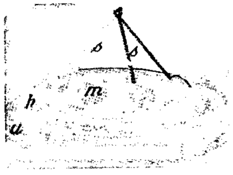
1. Електрофор: b кружок із живиці на доброму провіднику u; m металевий кружок на ізолюючих шовкових шнурках s.
