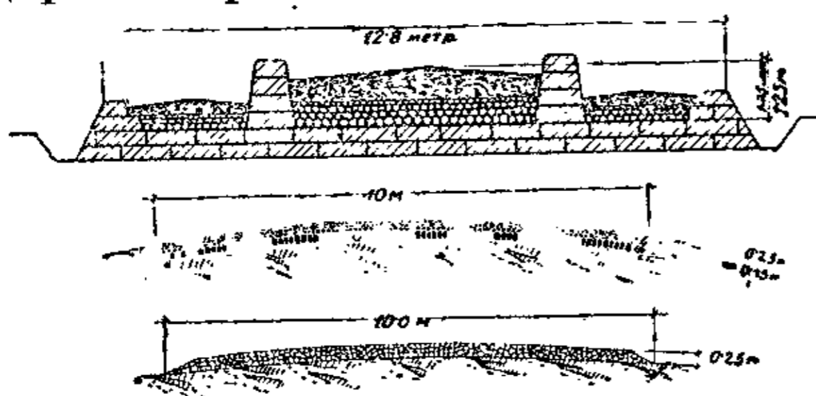
Дорога. Переріз: 1) римської д., 2) д. Трезагє, 3) д. Мек Адама.
