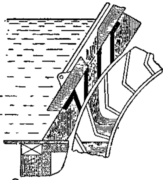
Середньоналивне колесо (частина).
