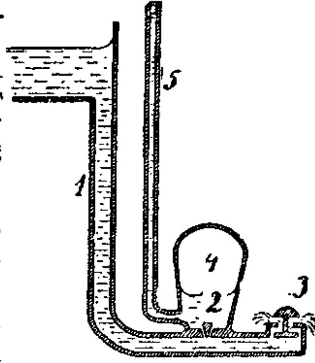
Гідравлічний таран Монгольф'єра: 1. рура, 2 і 3. затички, 4. збірник, 5. рура.
