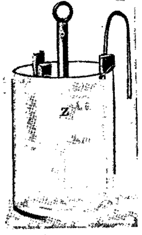
4. Гальванічна ланка: p олов'яна плита, z цинковий обруч.
