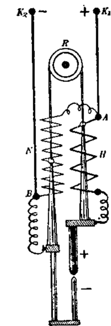
Дугова лампа [регулятор] N і H дротяні намотки, якими проходить головна (H) і побічна (N) електр. струя; R кружальце, на якому висять вугляні палочки; K 1 і K 2 електроди.
