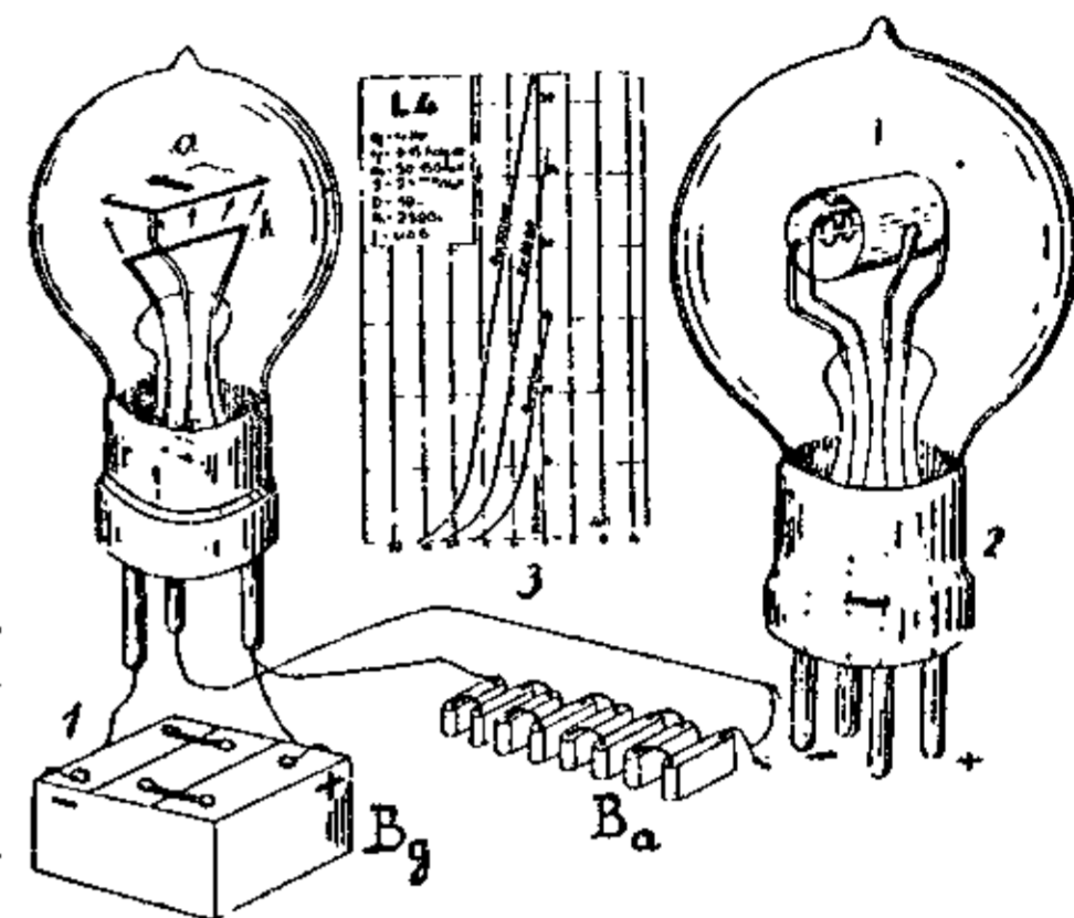
Електронні лампи: 1. діода, 2. тріода зі складовими частинами, 3. характеристика. V_a — анодна батарея, V_g — жарова батарея, а — анода, к — катода.
