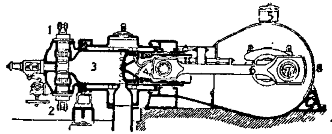
Двигун Дізеля. 1 і 2. вентилі, 3. циліндер, 4. толоч, 5. оливарка, 6. тягло, 7. корбовий вал, 8. охорона.
