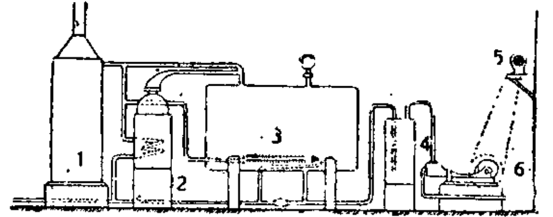
Паровий дезинфектор (схема). 1) Паровий котел, 2) котел з формаліною, 3) дезинфекційна скриня, 4) порожній котел, 5) двигун, 6) смок (помпа).
