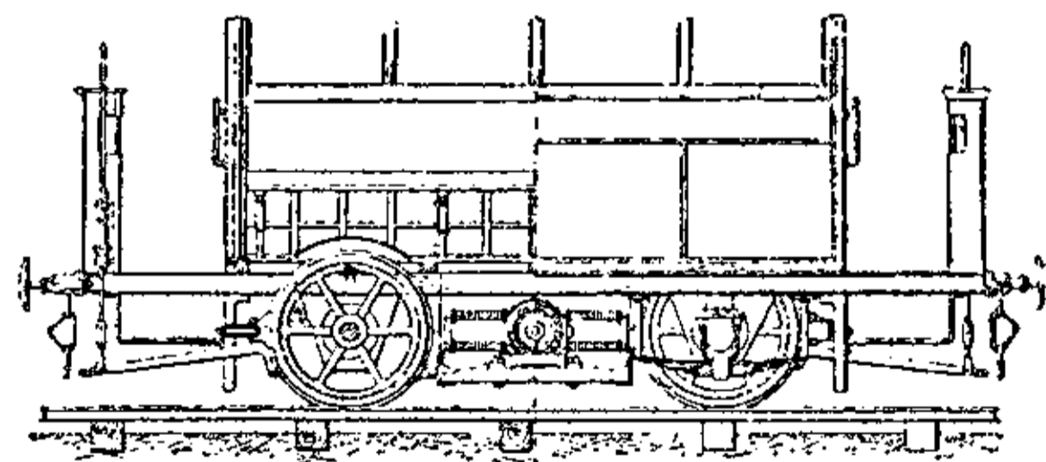
Електр. трамвай [схема спідньої частини возу].
