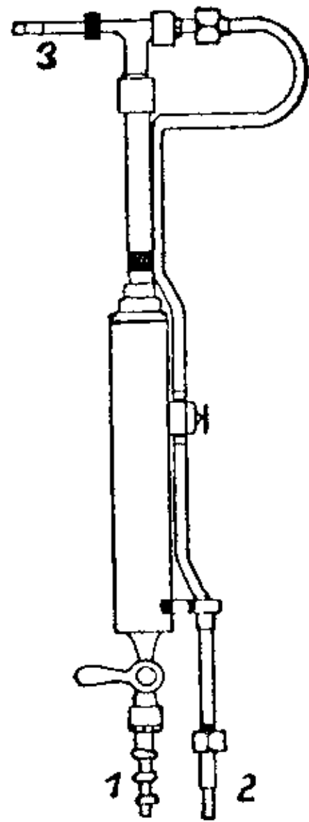
Автогенний прилад. 1. цівка, якою доходить водень або ацетилен; 2. цівка, якою доходить кисень; 3. пальник.
