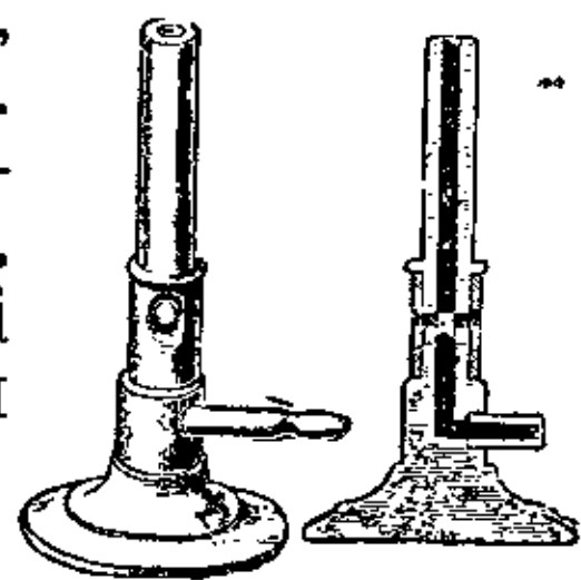
Пальник Бунзена.
