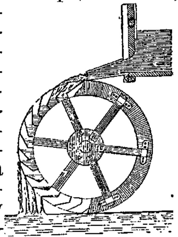
Верхоналивне колесо.
