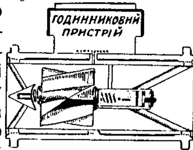
Вольтмана водомір до мірення кількості й шкорошти води.
