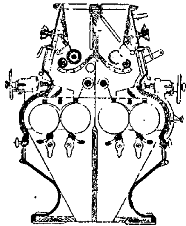
Вальцевий станок.
