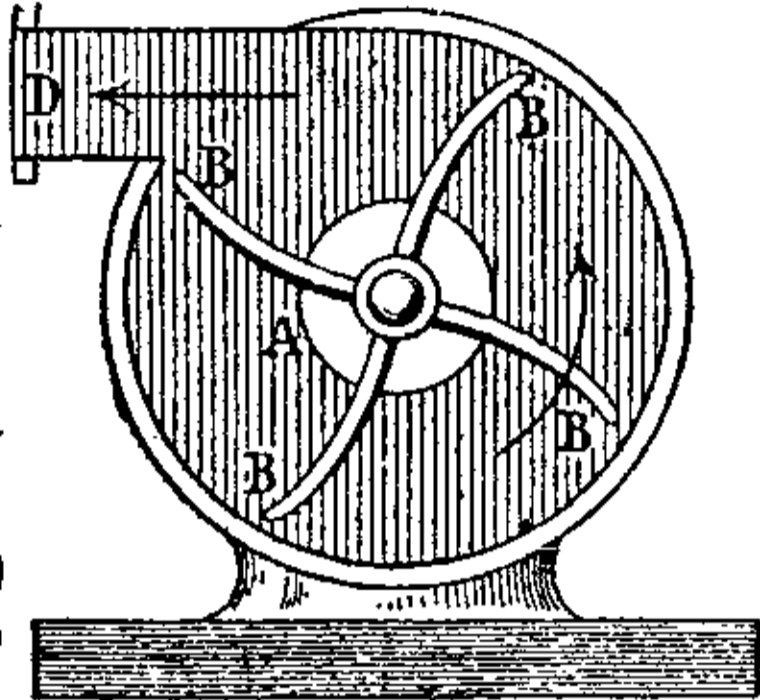
Вентилятор.
