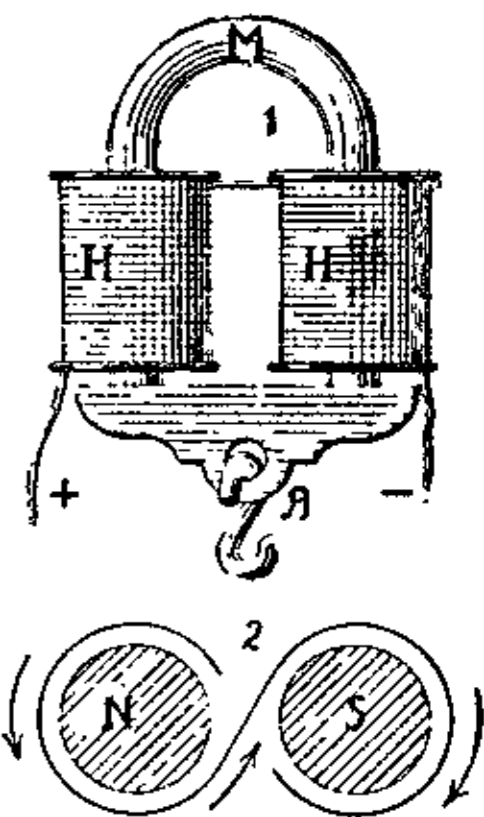
Електромагнет, 1) М — підковисто зігнений прут м'якого заліза; НН — намотки дроту, Я — якор; 2) попер. перекрій бігунів електромагнету, стрілки вказують напрям намоток, N — бігун півн., S — бігун півд.
