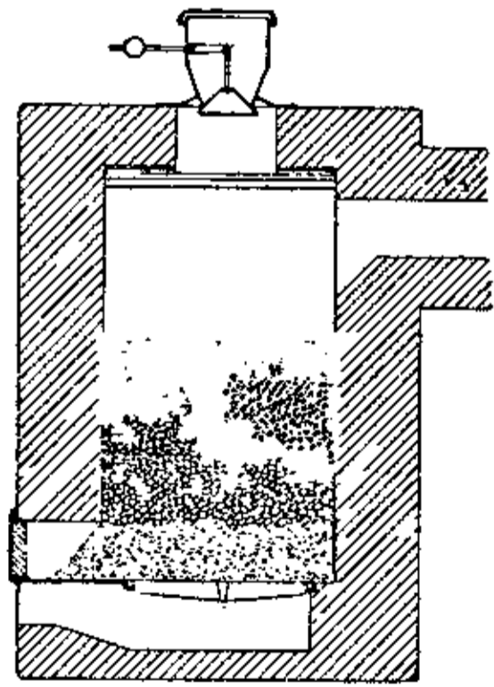
Газогенератор.
