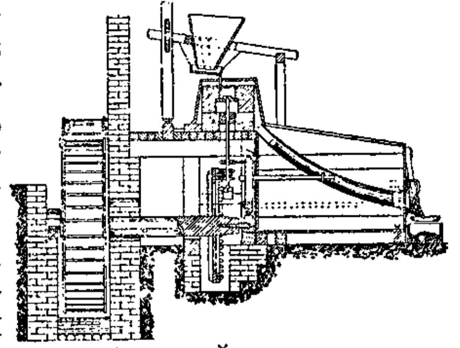
Водяний млин.
