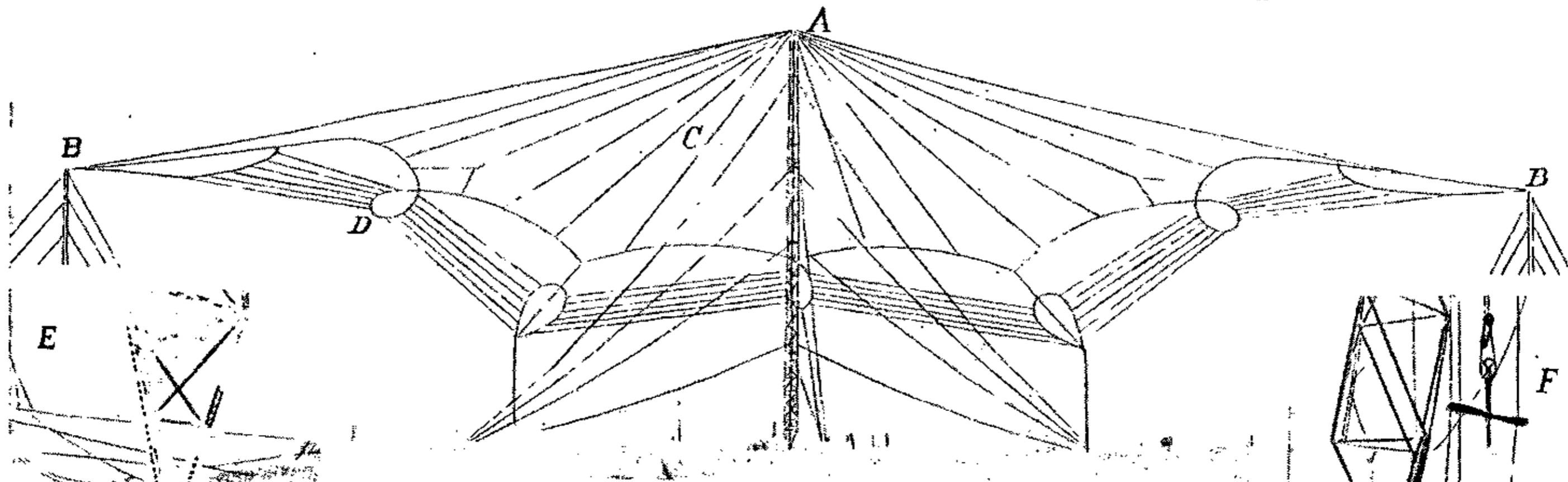
10. Уклад антен великої іскрової стачії в Айльвезе: A головна вежа (250 м. висоти); B 6 побічних щогол 122 м. висоти, віддалених 460 м. від головної вежі; C проміниста антена; D перстенева антена; E (наліво) підстава головної вежі; F (направо) підстава бічної щогли з тягарем до патиження антен.
