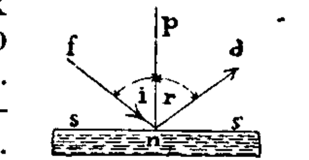
Горішній рисунок: відбивання хвилі; долішній: відбивання пружистої кулі.
