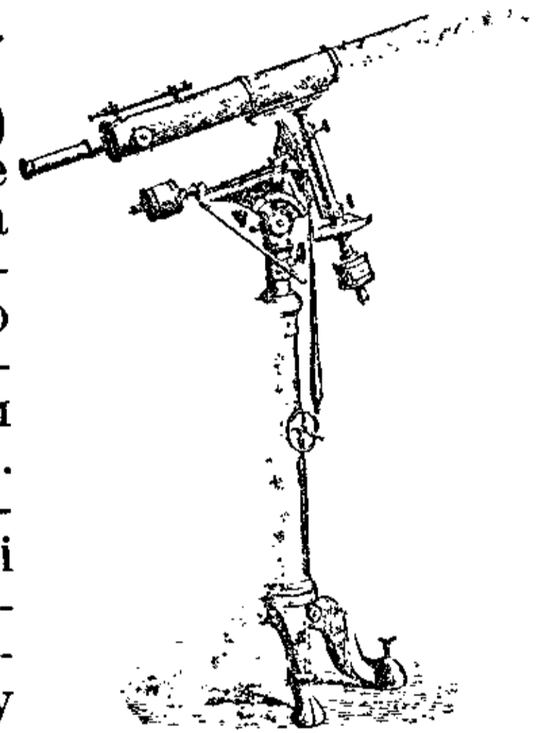
Екваторіал.
