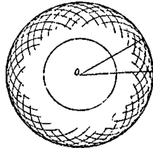
Закон Гойхенса: Хвиля, представлена більшим колом, є вислідною безлічі другорядних хвиль, яких осередки є на попередній хвилі.
