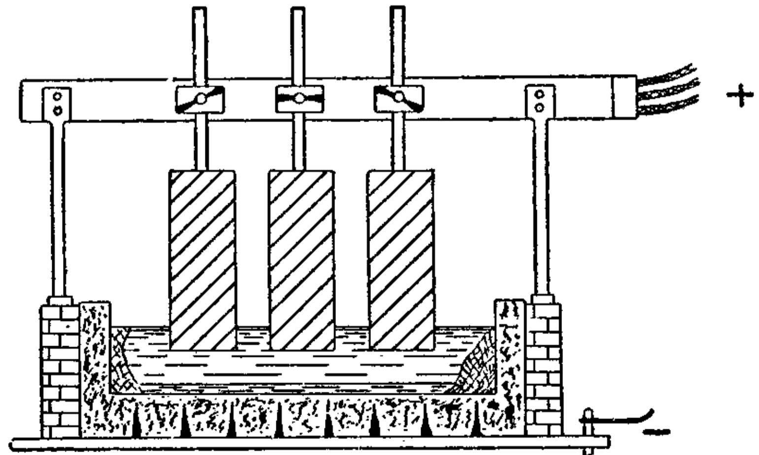
Піч Герульта (Heroult)
