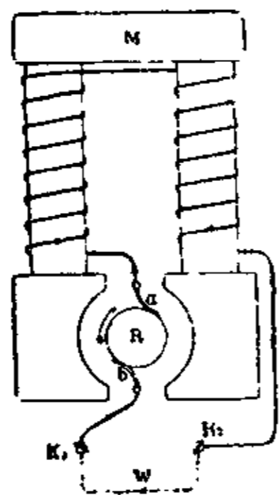
Схема динамомашини. М — електромагнет, R — перстень, а b — щітки, K 1 , K 2 — бігуни, W — зовнішній провідник, яким пливе електр. струя.
