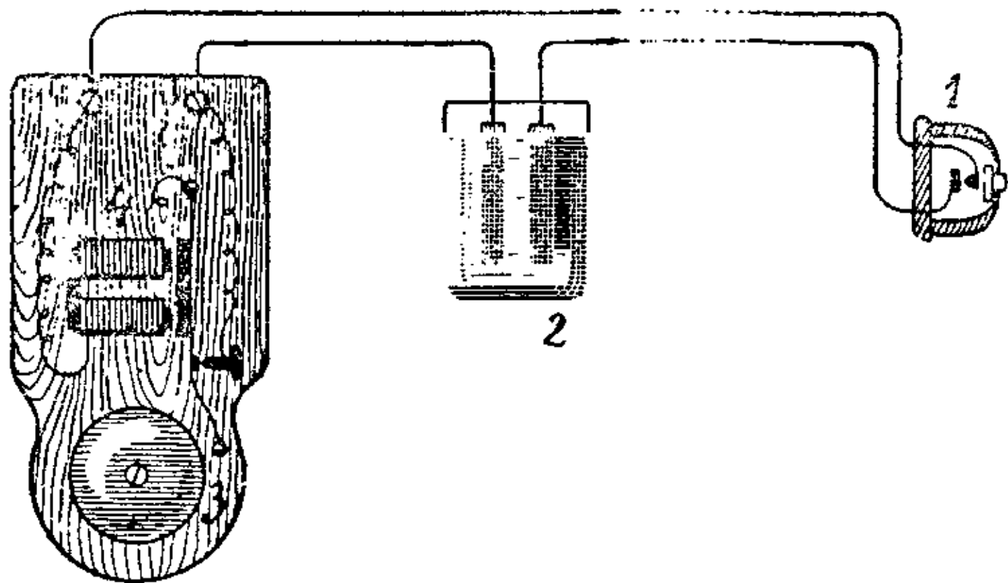
Електр. дзвінок [схема]: 1. гудзик до натискання, 2. гальванічна ланка, 3. дзвінок, 4. електромагнет.
