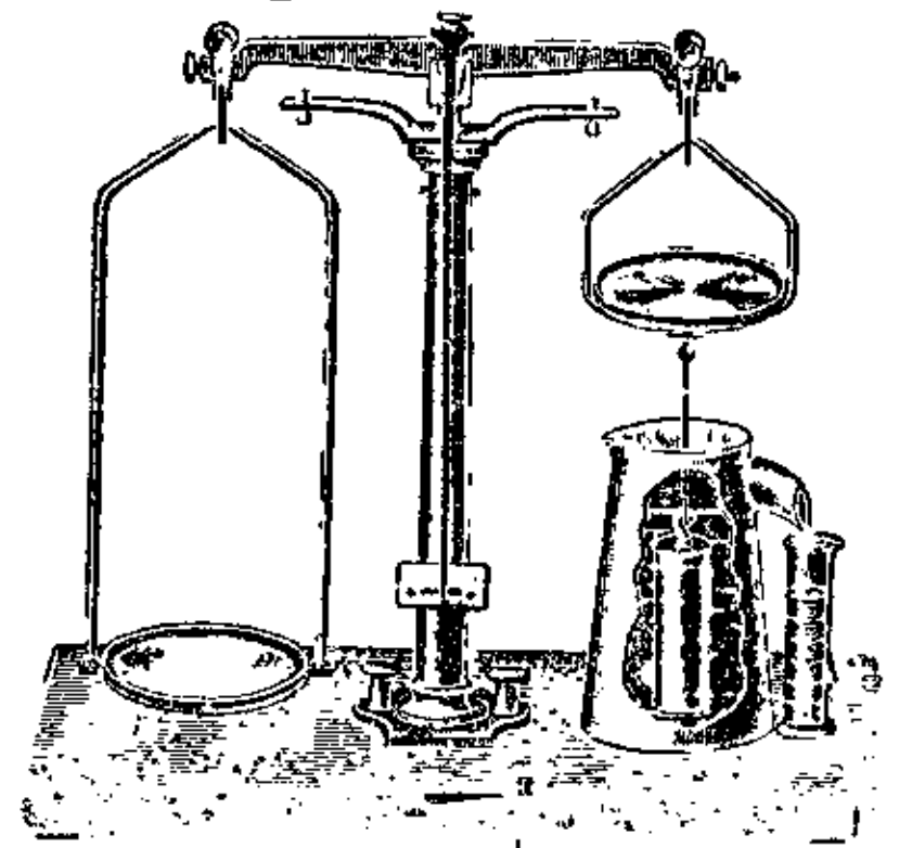
Вага до мірення взгону.
