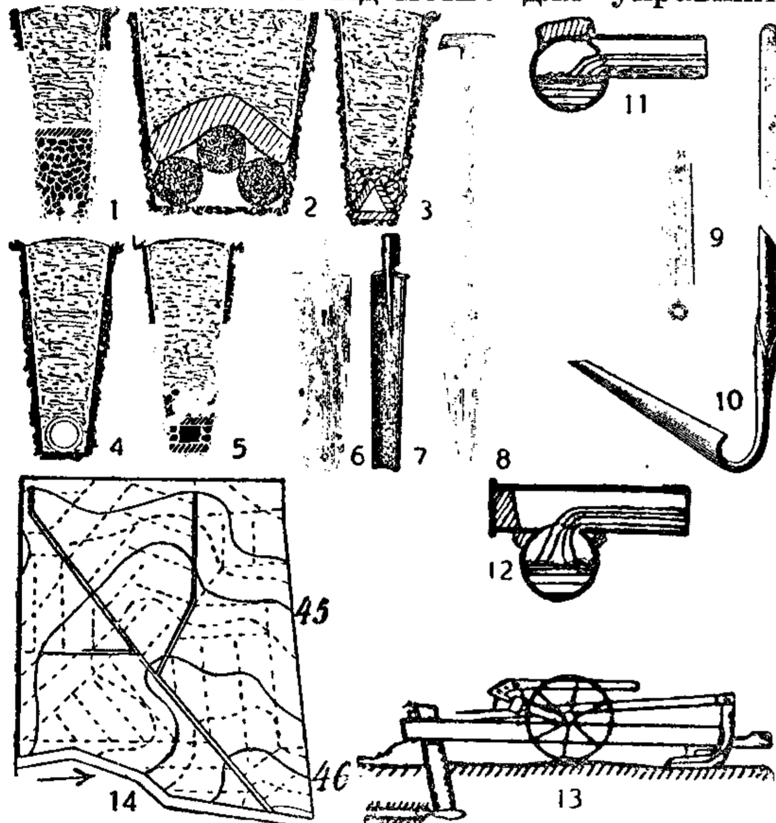
Дренаж. 1-5 переріз критих ровів, 6-10 приладдя до копання і чищення ровів, 11. споєння дренажних рур із боку, 12. згори, 13. плуг до дренажу ґрунту, 14. план відводнення мокрого ґрунту.
