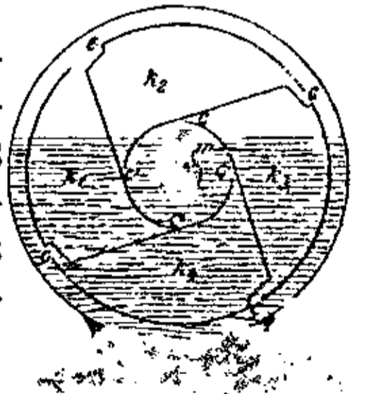
Газомір, k 1 —k 4 комори; c 1 —c 4 отвори; t—цівка, якою доходить газ.
