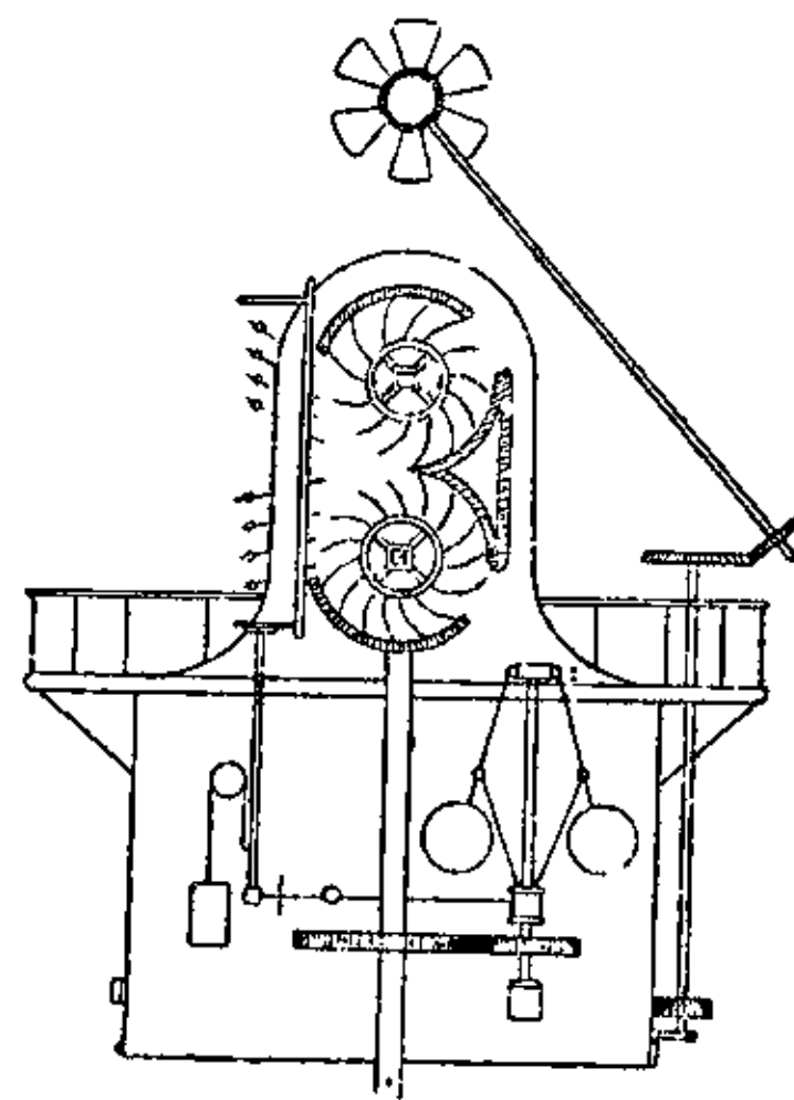
Вітряна турбіна.
