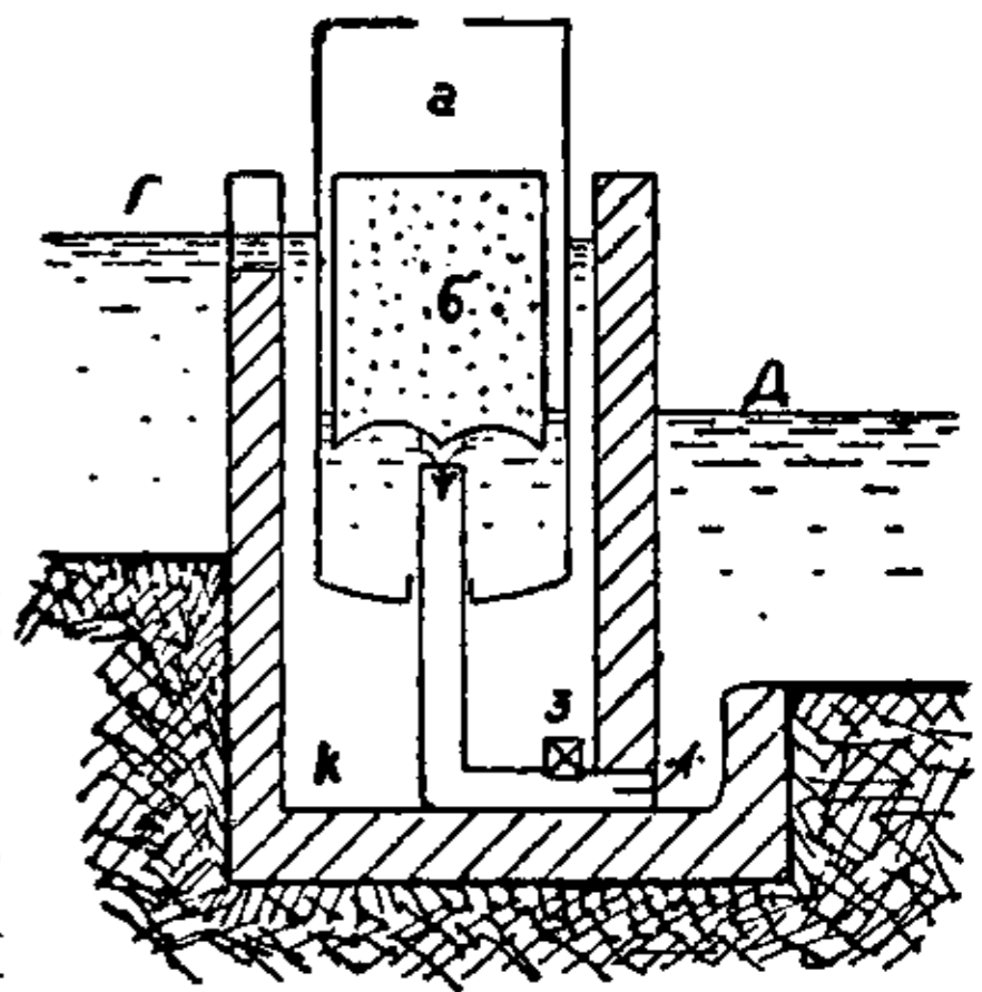
Аквапульсор. г — позем' горішн. збірника; д — позем' дол. збірника; к — шахта, а — пливак, б — затичка горішня, з — затичка долішня.
