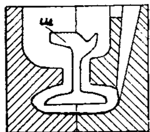
Сплювання шини алюмінотермією: ж = термітове залізо, ш = шина.
