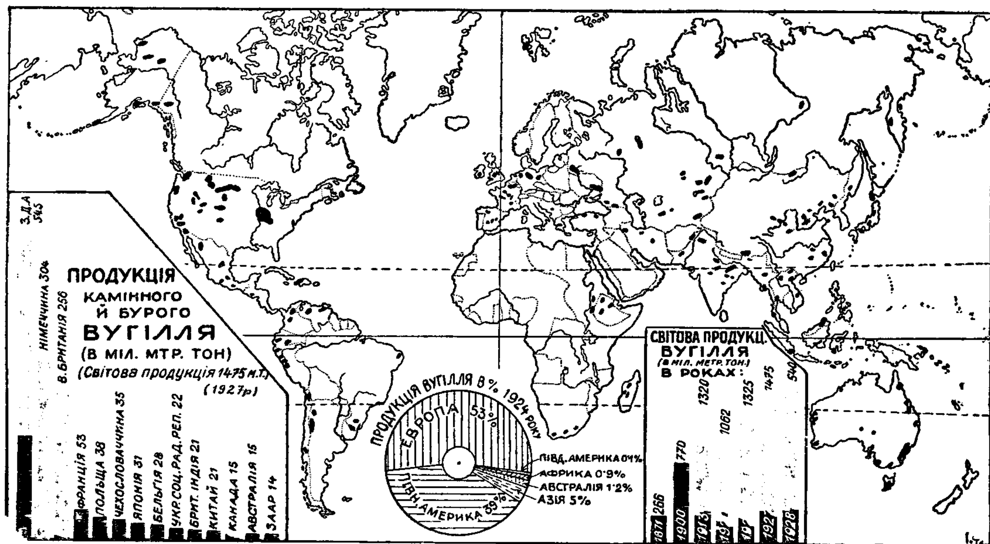
Вугілля (чорні цятки означають поклади вугілля).
