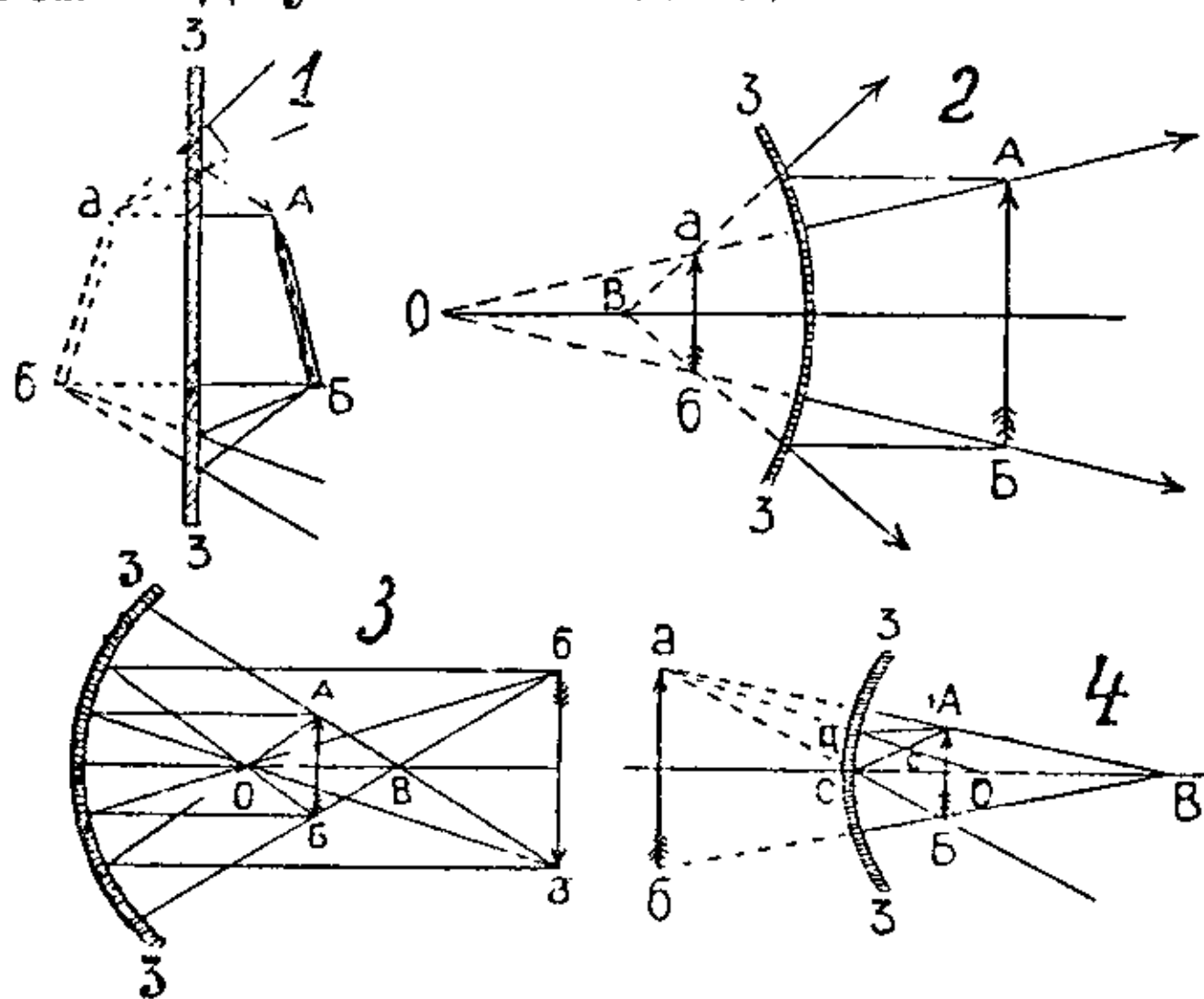
Дзеркало: 1. плоске дз., 2. вигнуте дз., 3. і 4. вгнуте дз. ЗЗ — дзеркало; АБ — предмет; аб — образ; О — в 2 осередок, в 3 і 4 огнище; В — в 2 огнище, в 3 і 4 осередок.
