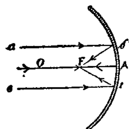
Головний промінь. OFA гол. промінь. AF відбитий гол. пром.; F огнище, аб, вг побічні пром.; бF, гF відбиті поб. пром.
