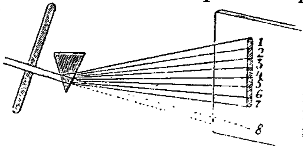
Дуговина. Промінь розщеплений на краски від фіялкової (1) до червоної (7); 8 місце, де впало б проміння, колиб не було призми.
