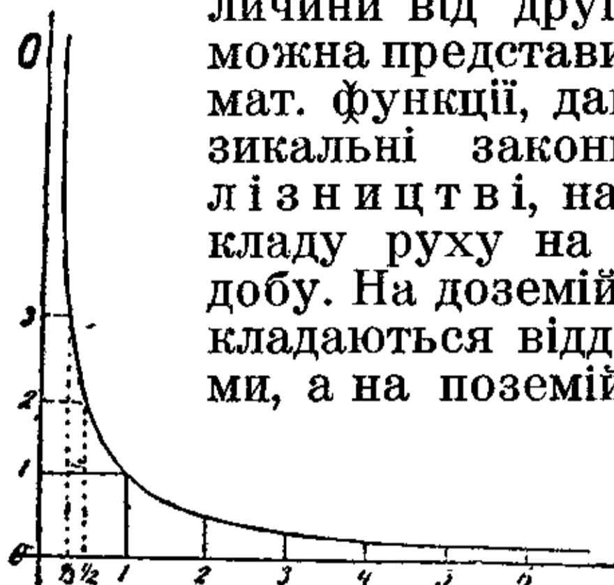
Графікѳн: зображує закон Бойль-Маріота; на доземій лінії відтинаємо величини об'єму (o), на поземій тиснення.
