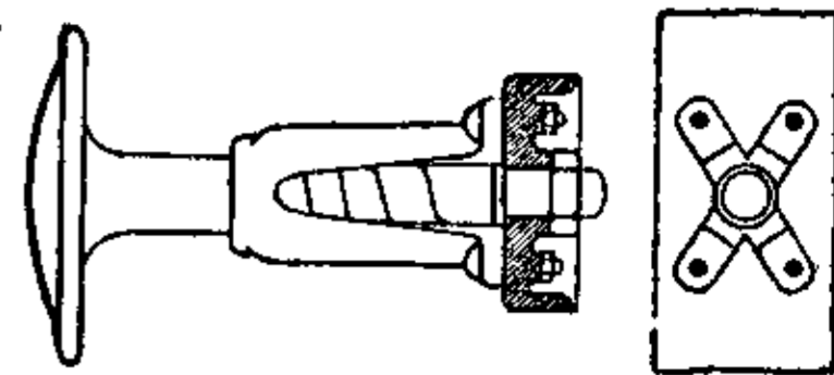
Буфер.
