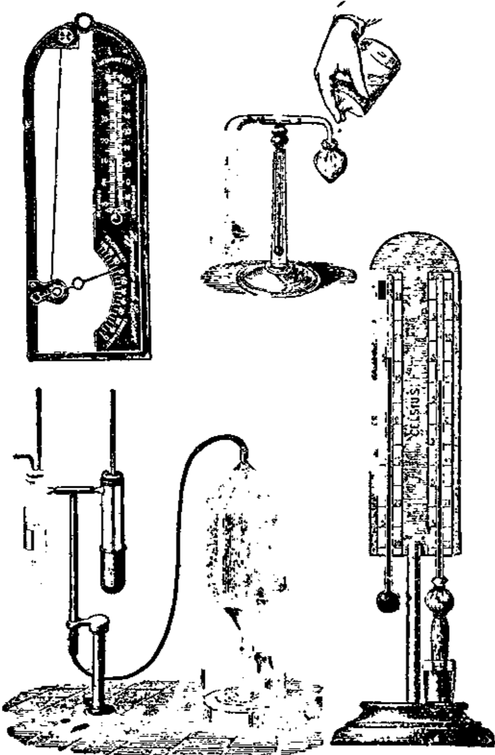
Гігрометри. Вгорі, від ліва: г. Соссюра, Данієля; вдоли, від ліва: г. Реньольта, психрометр Августа.
