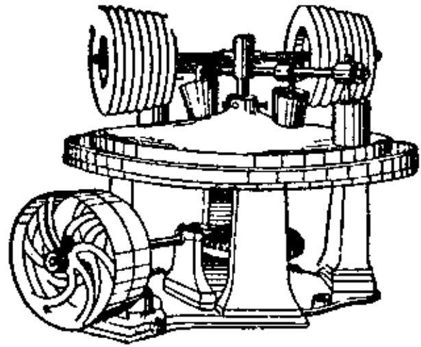
Глиняне виробництво: прилад до мішання глини.
