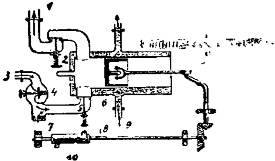
Газовий вибуховий двигун Отта (нарис). 1. рура, якою виходить газ, 2. вентиль, 3. рура, якою входить газ, 4. жарова рура, 5. рура, якою проходить газ змішаний з повітрям, 6. вентиль, 7. рура, якою входить повітря, 8 і 10. вал до керування вентилями, 9. рура, якою допливає холодна вода.
