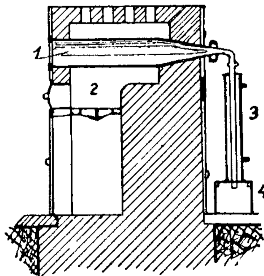
Піч до амальґамування. 1. Збірник (реторта), де працюється руда з ртуттю; 2. огнище; 3. холодильник; 4. збірник з ртуттю.
