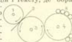
Офсетова машина (схема): 1, 3, гумові вальці, 2 папір, 4, валець з матрицею, 5, валець, що піднімає, 6, що розтирають фарбу.
