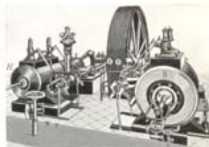
4. Машина з бічним уламковим циліндром, із вертикальним випуском пара; Н циліндр із високим тисаком, X циліндр із низьким тисаком.
