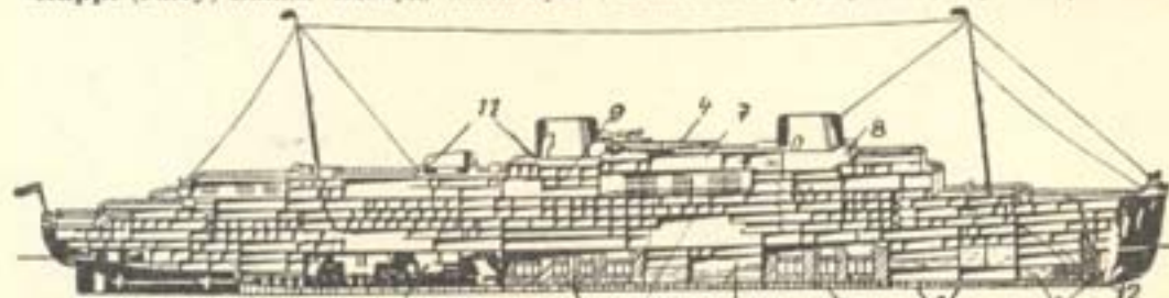
Перекріз сучасного пароплаву. 1. машини, 2. кіліни, 3. куліна, 4. літан, 5. збірники води, що зливаються коливання корабля, 6. подвійне дно, 7. ресторан, 8. місце команданта, 9. бездротний телеграф, радіо, телефон, 10. ліжусові помешкання, 11. змагові площі, 12. гаражі для авт. Малі перегородки це каюти.
