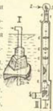
Перископ відвідного човна (1) його нарис (2) 1. сталева труба (15-20 см. проміру), 2. проміня заломлюється в призм (3), так що переходить через кілька сочок (4) і призм (5) та відбите в призм (5) виходить отвором (6).
