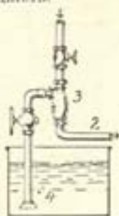
Ін'єктор 1) — вгорі — паровпусна труба. 2. паровпусна труба. 3. ін'єктор. 4. смон. що ссе воду.
