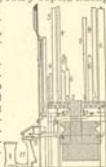
Органи (перезрій): 1. міх, 2. продувальний рукав, 3. повітрогон, 4-7. дудки; 4. отаєрті металеві, 5. отаєрті дерев'яні, 6. заверті, 7. з'єднанні, 8. клавіатура, 9. соло'яні рукави, 10. рукава для реєстрування, 11. педалі.
