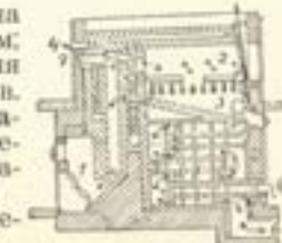
Крематорія (перепр.). 1. огнище, 2. місце сжеле- ннн, 3. попельнице, 4. рури, якими прозодить повітря, 5. рури, якими прозодить газл, 6. ви- від до конина, 7. вікон- це, яким можна огляда- ти сжелення.
