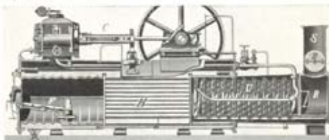
6. Шестигонний: F шестигонний, H горизонтальний циліндр, G вертикальний, в димовий кошик, B тисак, D рухома шина, С шина з бічним уламковим циліндром.
