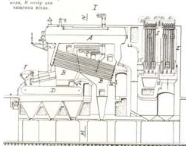
3. Котел Штайнхеймера:
