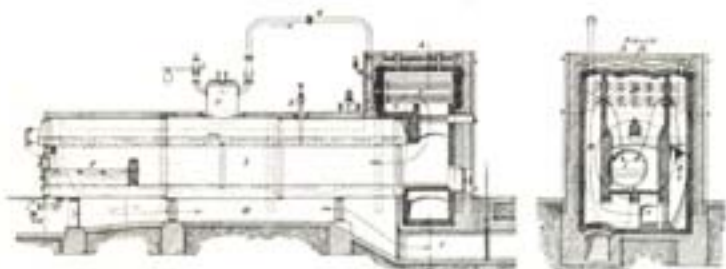
2. Котел з одним горизонтальним трубою з перегородками (похилою і горизонтальною перегородками A-B ):
