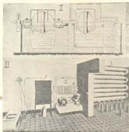
Самочина (I) й машинна (II) заводська молока; 1. компресор, 2. кондензатор, 3. рефригатор.
