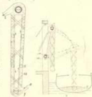
Норія: 1. схема нерухомої н.і черпаки (а) черпають збіжжя (в) і піднімають його вгору та здійснюють отвором (г), б — ложки; 2. рухома норія.
