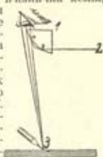
Камера люцида: 1. чотиригранна шкляна призма, 2. промінь, що виходить з предмету, або краєвиду, а. 3 — відбитий промінь, 3. образ предмету або краєвиду.
