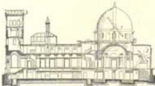
Астрономічна обсерваторія (черес): 1. рефрактор, 2. теліограф, 3. вежа.
