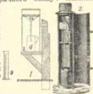
Омброметр. 1. У вальці — 2. уміщена посудина — 3. куди падає дощ і співає до посудини — 4. Кількість опадів міряно мензурою — 5. 2. Гельмановий регистраційний омброметр (омброметр) що сам зазначає кількість води.
