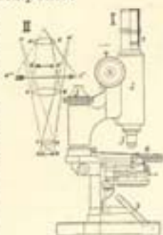
Мікроскоп. I. нарис. 1. окуляри, 2. туба, 3. об'єктив, 4. шруба до приблизного наставлювання м., 5. шруба до докладного наставлення, 6. підставка на предмет, під нею кондензор і 7. дзеркало для освітлення предмету; II. вияснення повстання образів в м., HO, FE сочиня окуляру, CD сочиня об'єктиву, AB малий предмет, A'B' образ збільшений сочною HO, A''B'' знову збільшений образ сочною FE.
