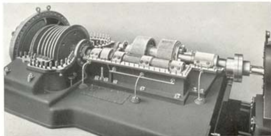
7. Парова турбіна (виготовлена компанією А.А. Том. Листопад Шпроберт) що має три парні шари для рухомих шин з лопатками, в посередній шині зубчастий вал для перетворення швидкості обертів турбіни (3000 на хв.) на меншу швидкість генератора (918 на хв.).
