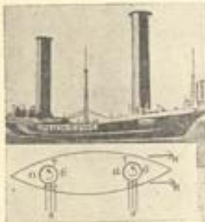
Верхні: флетнерівський роторний корабель „Бухан“. Вдолі: схема роторного корабля. тт — труби, стрілка всередині вказує напрям обороту, а, б — розвіджене й згущене повітря, в — напрям вітру, н — напрям руху корабля.
