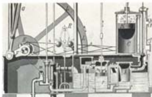
1. Парова машина Нотта (1884).
