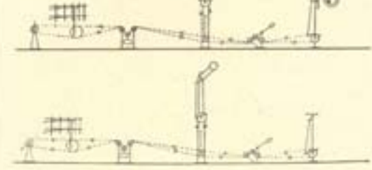
Схема семафору. Вгорі зал. семафори, наставлені на знак, що шлях замкнений, вгорі семафори, наставлені на знак, що шлях вільний для проїзду.
