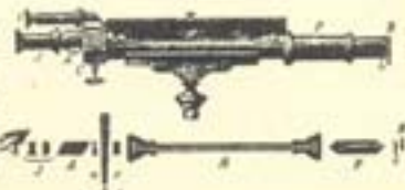
Сахариметр. В — плита, крізь яку проходить промінь, L — збиральна сочка, P — призма, що поляризує світло, R — пробна труба, а, б, с — внаслідок призма, с — компензатор, А — призма Нікола, тзв. аналізатор, J — малий дальновід.
