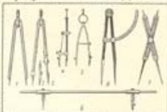
Циркул: 1. відмірювати віддалі, 2-3. рисувати арки й кола, 2. олівцем, 3. тушем або чорним, 4. рисувати малі кола (гзв. нульовий ц.), 5. відмірювати довжину й рисувати кола, 6. відмірювати кути, 7. редуційний, 8. рисувати великі кола (гзв. штанговий).
