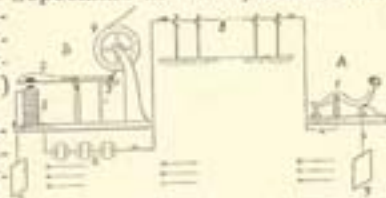
Схема телеграфу. А — станція надання, В — станція приймання. 1. стукач, 2. писальний прилад, 3. писальне, 4. паперова лента, що обертається при допомозі годинникового приладу, 5. електромагнет, 6. електр. ланка, 7. плати в землі, 8. дроти.
