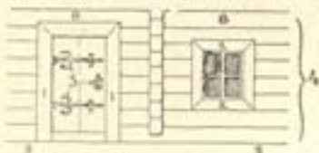
Частини укр. дерев'яної рубленої хати: 1. одвірні або лутки, 2. ослупи, 3. новані двері, 4. оструб, 5. підваліни, 6. правалі.
