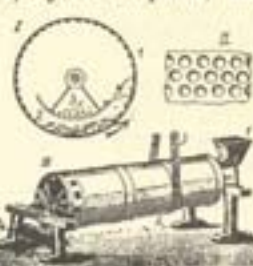
Трієр: 1. пережрій, 1. барабан, 2. прочищаче зерно, 3. замешчення; 2. частина стінки барабана з отворами; 3. цілий трієр, 3. отвір, куди висипають збіжжя, 2. барабан, 3. ремень, 4. отвір, куди виходить прочищене збіжжя.
