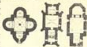
VI. Планки будів. XV-XVI в. в кін. XIV. в., Перемишлі 1460 й Кам'янці з кін. XV. 1. Сутківці, 2. Рыботицька посада, 3. Залужка.
