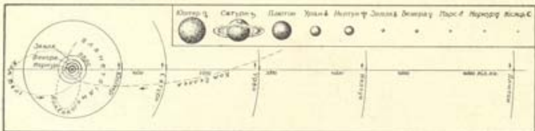
Сонячна система: дороги планет кругом Сонця; згорі планети уложені чергую, відповідно до величини.
