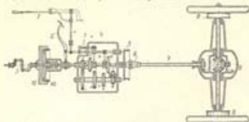
Самоходовий двигун: 1. валиць, 2. ступиць, 3. колінчатий вал двигуна, 4. коробка швидкості, 5. гальмове кружало, 6. сугаставний вал Кардана, 7. вал, 8. гальмове кружало, 9. задня вісь із диференціалом, 10. мазовки зі злученням.
